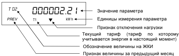
Рис. 2.3 Расположение информации на индикаторе
