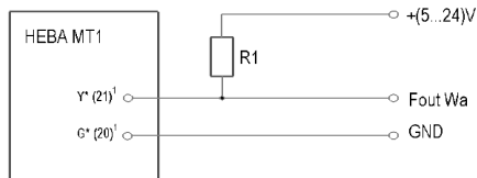
Схема подключения импульсных выходов счётчиков НЕВА МТ1
