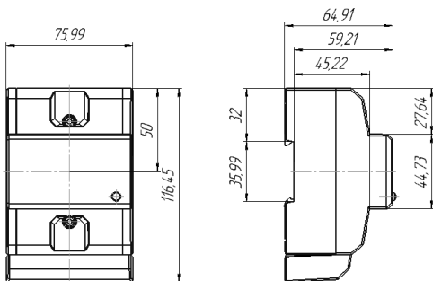
Внешний вид счётчиков НЕВА МТ 123
