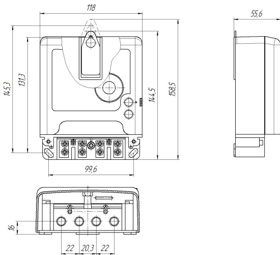
Установочные размеры счётчиков NEBA MT 11X
