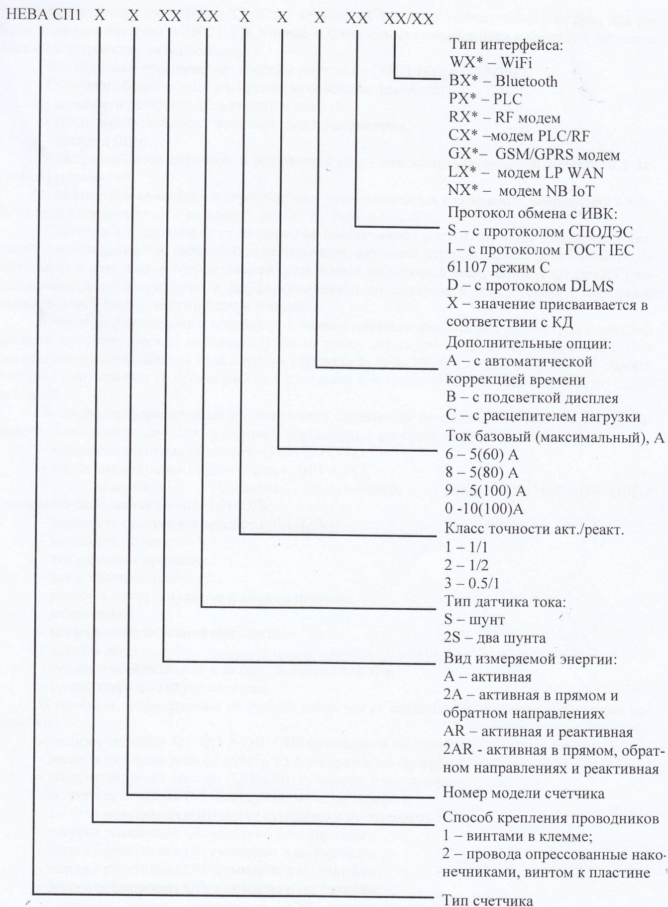
Рисунок 1 - структура условного обозначения счетчика
