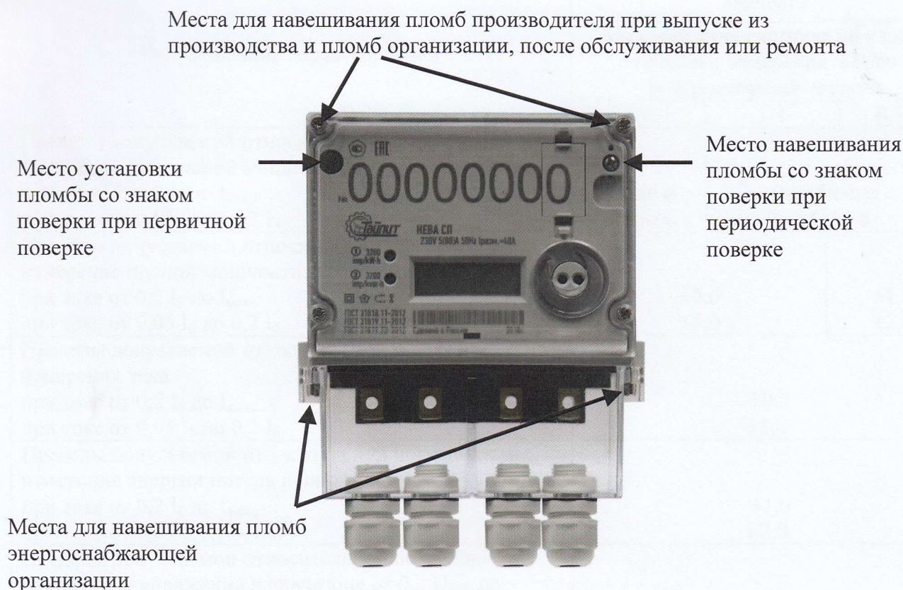
Рисунок 2 - Счетчик электрической энергии однофазный НЕВА СП1
