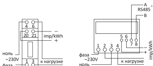
Схема включения счетчика НЕВА 102, НЕВА 105
