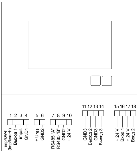
Схема подключения испытательных выходов счетчиков НЕВА СТ4ХХ
