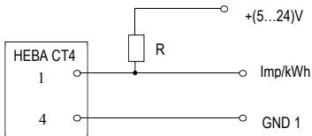
Рисунок 3 Подключение испытательных выходов счетчиков HEBA CT4
