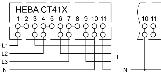
Схема включения счетчиков НЕВА СТ41Х непосредственно в сеть
