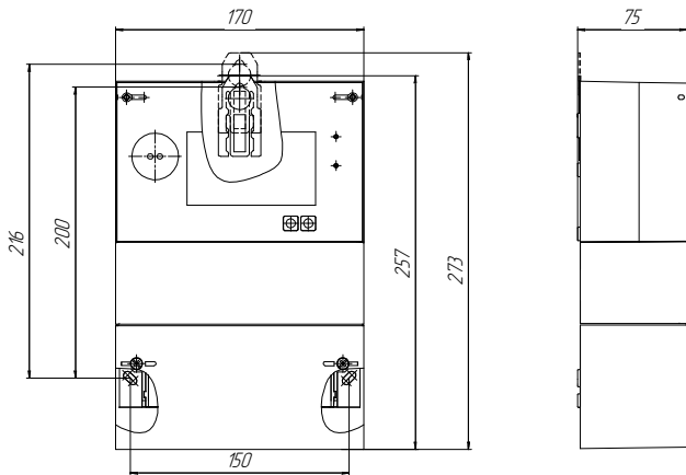
Внешний вид счетчиков НЕВА СТ4ХХ
