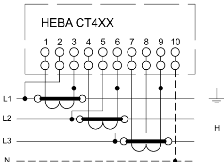
Схема включения счетчика HEBA CT4XX через трансформаторы тока в четырехпроводную сеть
