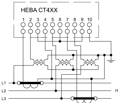
Схема включения счетчика HEBA CT4XX через два трансформатора тока и три трансформатора напряжения в трехпроводную сеть
