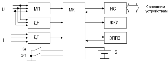
Рисунок 1.2 – Функциональная схема счетчика
