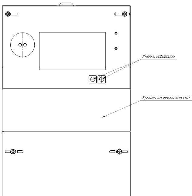
Внешний вид счетчиков НЕВА СТ4ХХ в сборе
