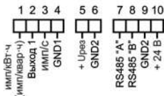
Схема подключения НЕВА СТ4ХХ без дополнительного модуля входов/выходов
