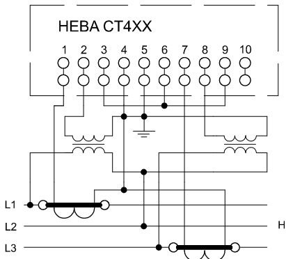
Схема включения счетчика HEBA CT4XX через трансформаторы тока и трансформаторы напряжения в трехпроводную сеть
