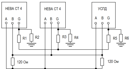
Рисунок 2.2 – Схема подключения счетчиков к интерфейсной линии EIA 485
