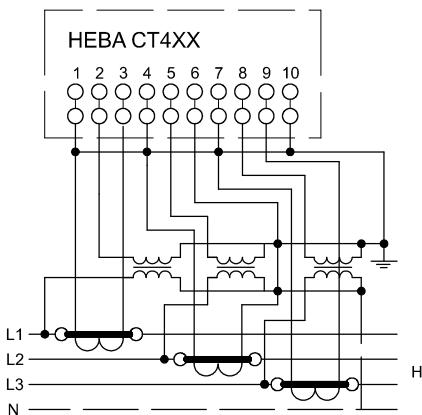
Схема включения счетчика HEBA CT4XX через трансформаторы тока и трансформаторы напряжения в четырехпроводную сеть
