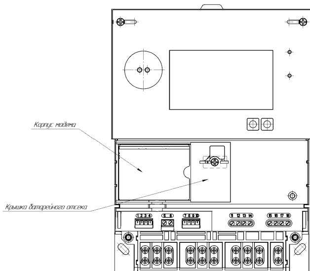
Внешний вид счетчиков НЕВА СТ4ХХ со снятой крышкой клеммной колодки
