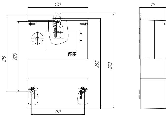
Внешний вид и размеры счетчиков НЕВА СТ4ХХ
