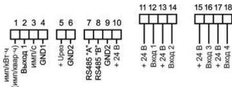
Схема подключения НЕВА СТ4ХХ с дополнительным модулем IO40
