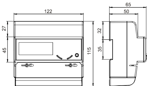
Внешний вид счетчиков НЕВА МТ32Х
