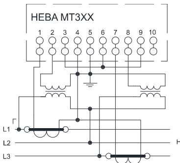
Схема включения счетчиков HEVA MT3XX через трансформаторы тока и трансформаторы напряжения в трёхпроводную сеть
