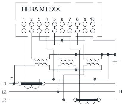
Схема включения счетчиков HEVA MT3XX через два трансформатора тока и три трансформатора напряжения в трёхпроводную сеть
