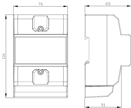
Внешний вид счётчиков НЕВА МТ 123
