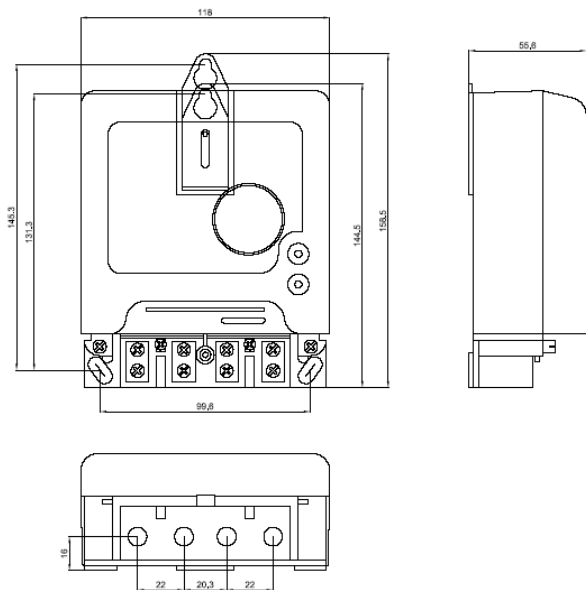
Установочные размеры счётчиков НЕВА МТ 11Х
