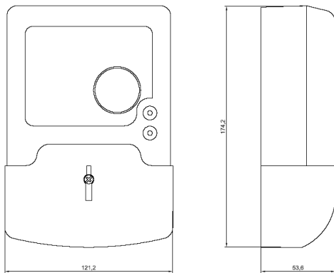
Внешний вид счётчиков НЕВА МТ 11Х
