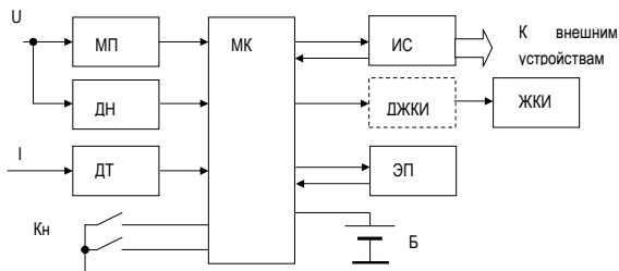
Рисунок 1 Функциональная схема счётчика.
