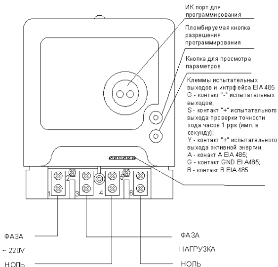
Схема подключения счётчиков НЕВА МТ 11Х
