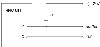
Схема подключения импульсных выходов
