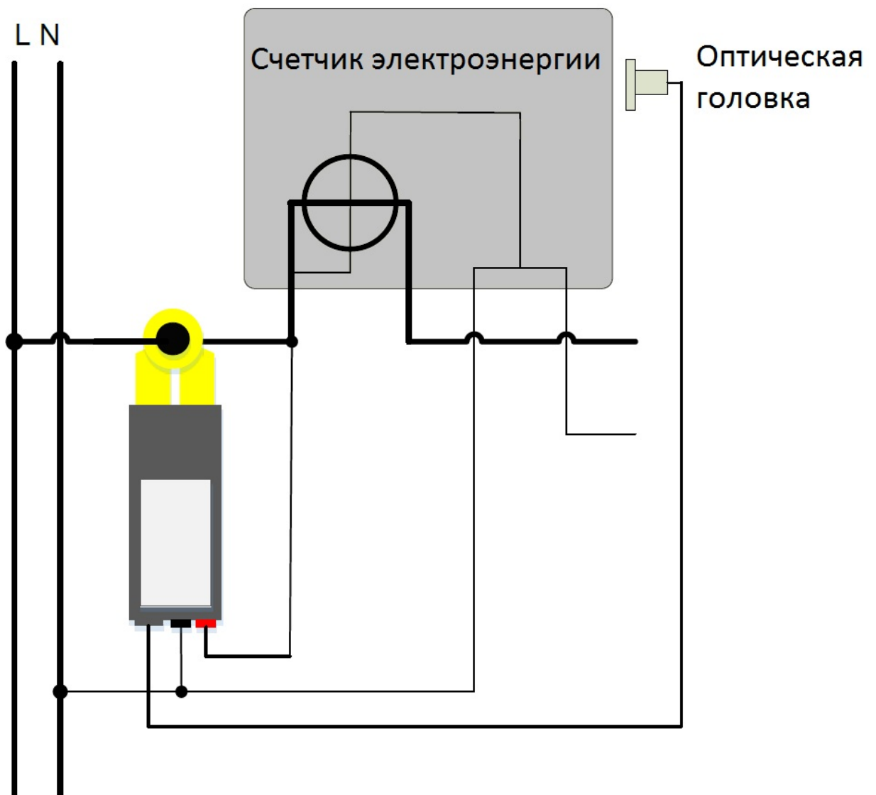
Рисунок 3.3. Схема подключения Прибора НЕВА-Тест 7203
